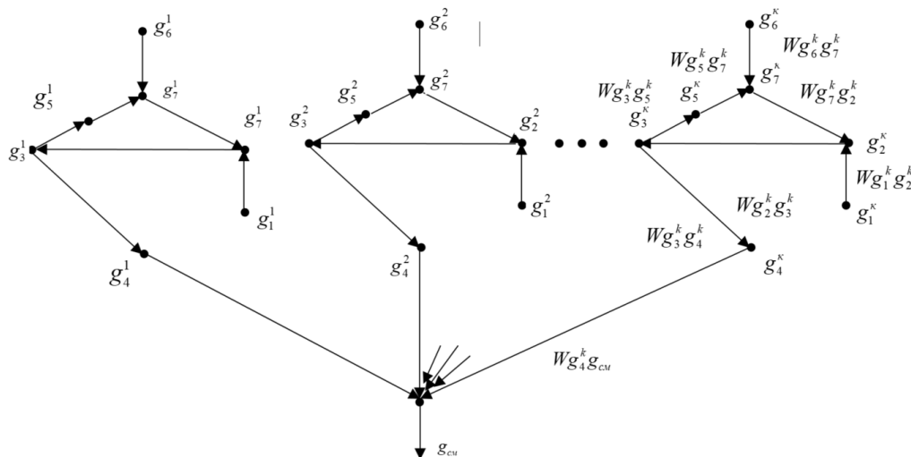
Рис. 3. Граф сигналів системи багатоконпонентного дозування при незв'язаному дозуванні
