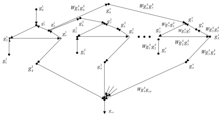
Рис. 4. Граф сигналу системи багатоконпонентного дозування матеріалів при зв'язаному з'єднанні дозаторів, коли головний компонент ведучий
